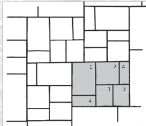
Unika-Verband VI / Unika pattern VI Römischer Verband / Roman pattern
