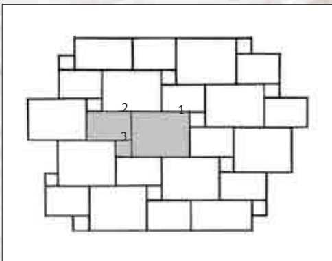
Unika-Verband III / Unika pattern III Römischer Verband / Roman pattern Achtung: Fugenabzug bei kleinem Format
